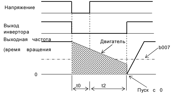
(пример 4) Выходная частота (время вращения двигателя) < b007
